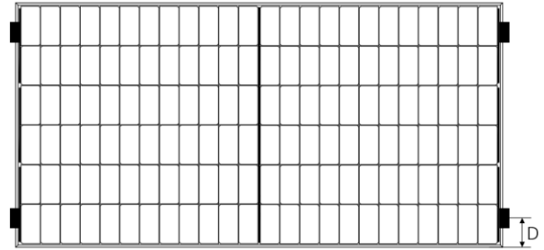
Fig. 6 Montaje con cuatro pinzas en el borde corto del marco
