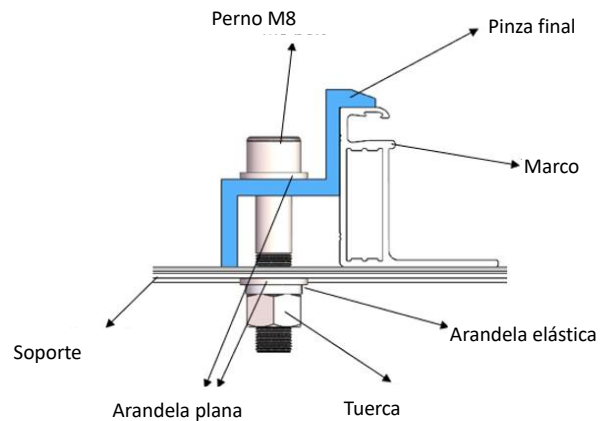
Fig. 9 Diagrama esquemático de instalación de pinza
