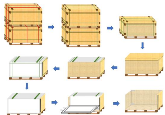
U型包装拆包步骤
