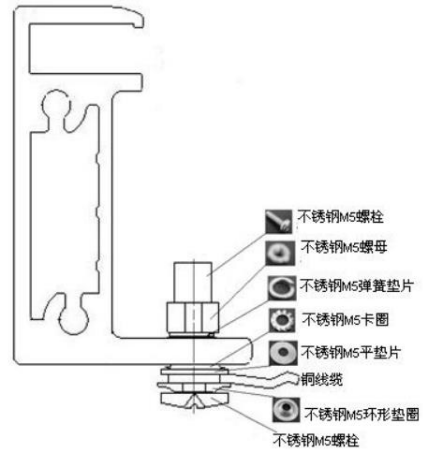
图 12 使用铜线缆将铝边框接地
