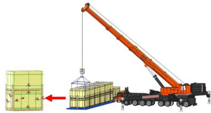
短边立式、U型包装吊车卸货示意图
