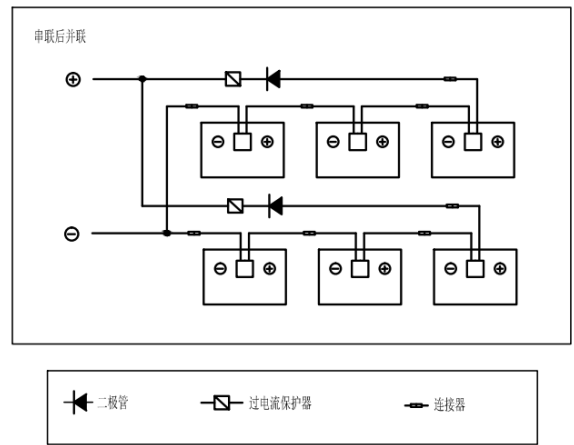
图 11 电联接示意图
